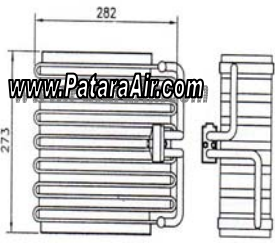
LANDCRUISER VX80,VX100 หน้า R-12,134A 06421
