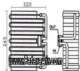
PREVIA R-12 ตู้หน้า 06430
